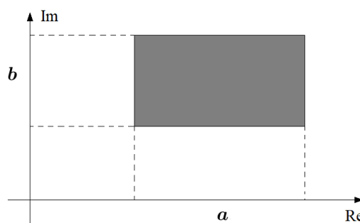
Рис. 2: Прямоугольный комплексный интервал
